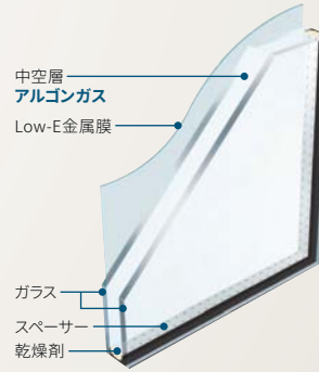
Low-E 複層ガラス(ガス入り)
