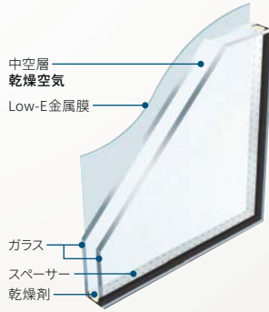
Low-E 複層ガラス(遮熱)
